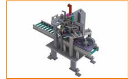
Prüfstation zur Vermessung der Betätigungs-kräfte und der Funktion einer Fußfeststell-bremse Test station for the measurement of the actuation forces and the function of a foot-operated parking brake
